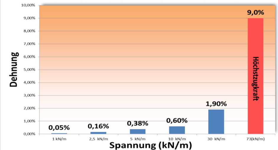
Dehnung bei spezifischen Spannungen 70000 S7L, 70000 H7L, 70000 T7L, 70000 T7L+, 70000 Q7L
