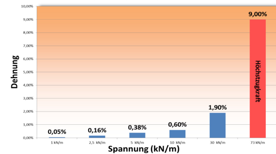
Dehnung bei spezifischen Spannungen 70000 SL, 70000 HL, 70000 TL, 70000 TL+, 70000 QL
