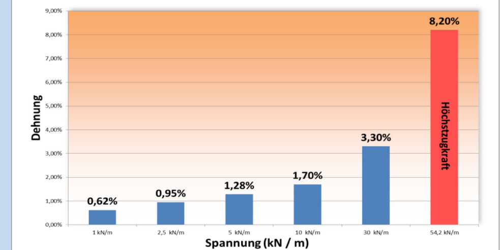
Dehnung bei spezifischen Spannungen 60000 SL, 60000 HL, 60000 TL, 60000 TL+, 60000 LL, 60000 QL
