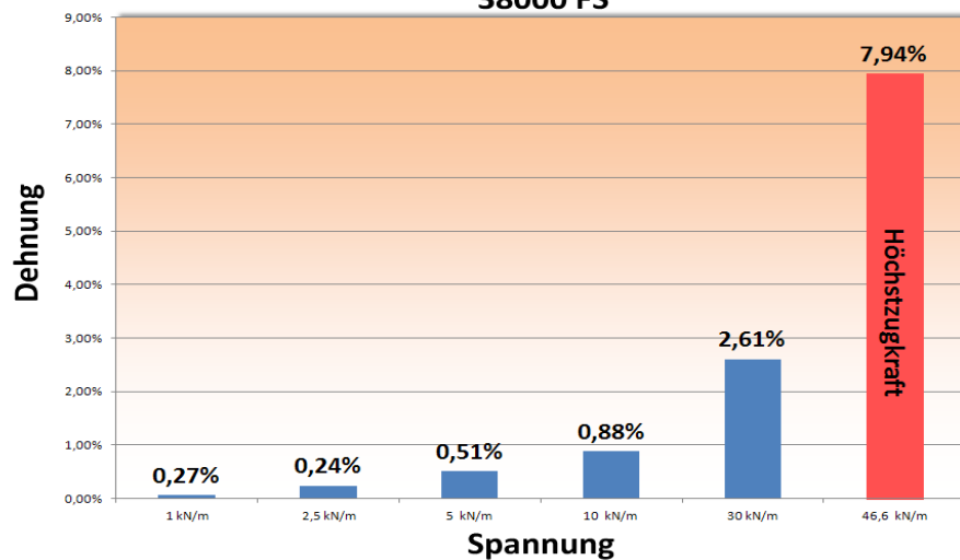
Dehnung bei spezifischen Spannungen 38000 FS
